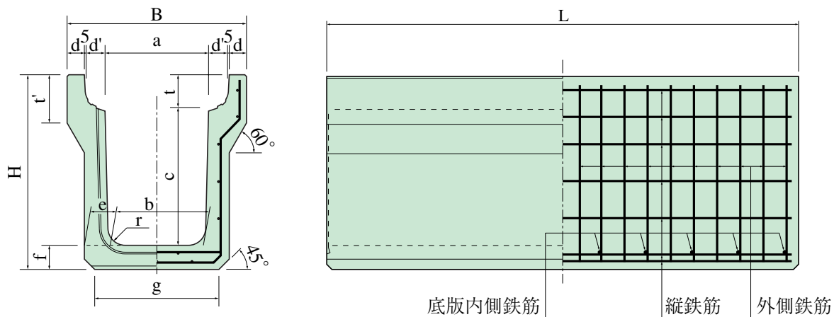
側溝本体形状図
