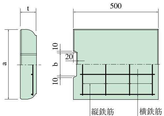
ふた形状図
