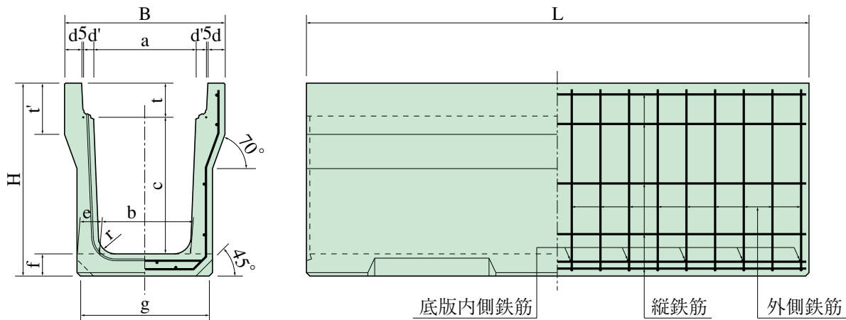
側溝本体形状図
