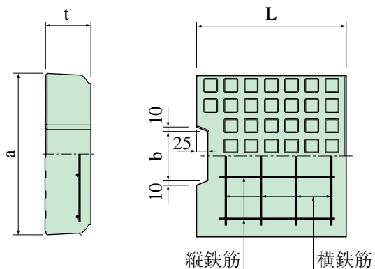
ふた形状図
